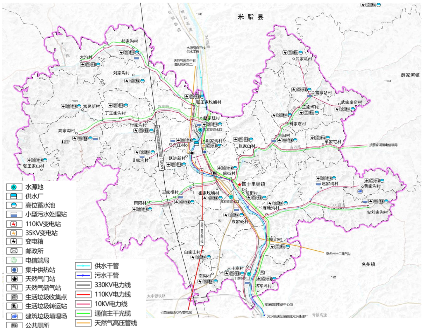
市政基础设施规划图
