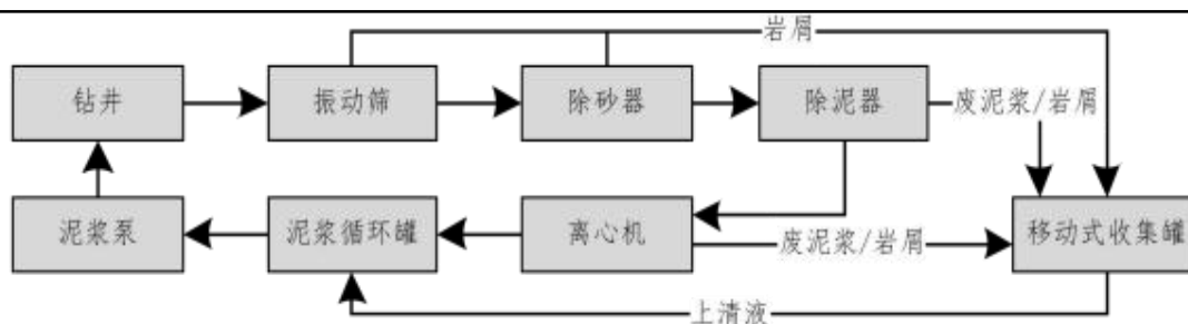
图 2-5 泥浆闭路循环系统示意图
