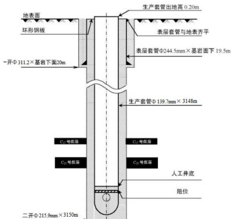
图 2-6 井身结构示意图
