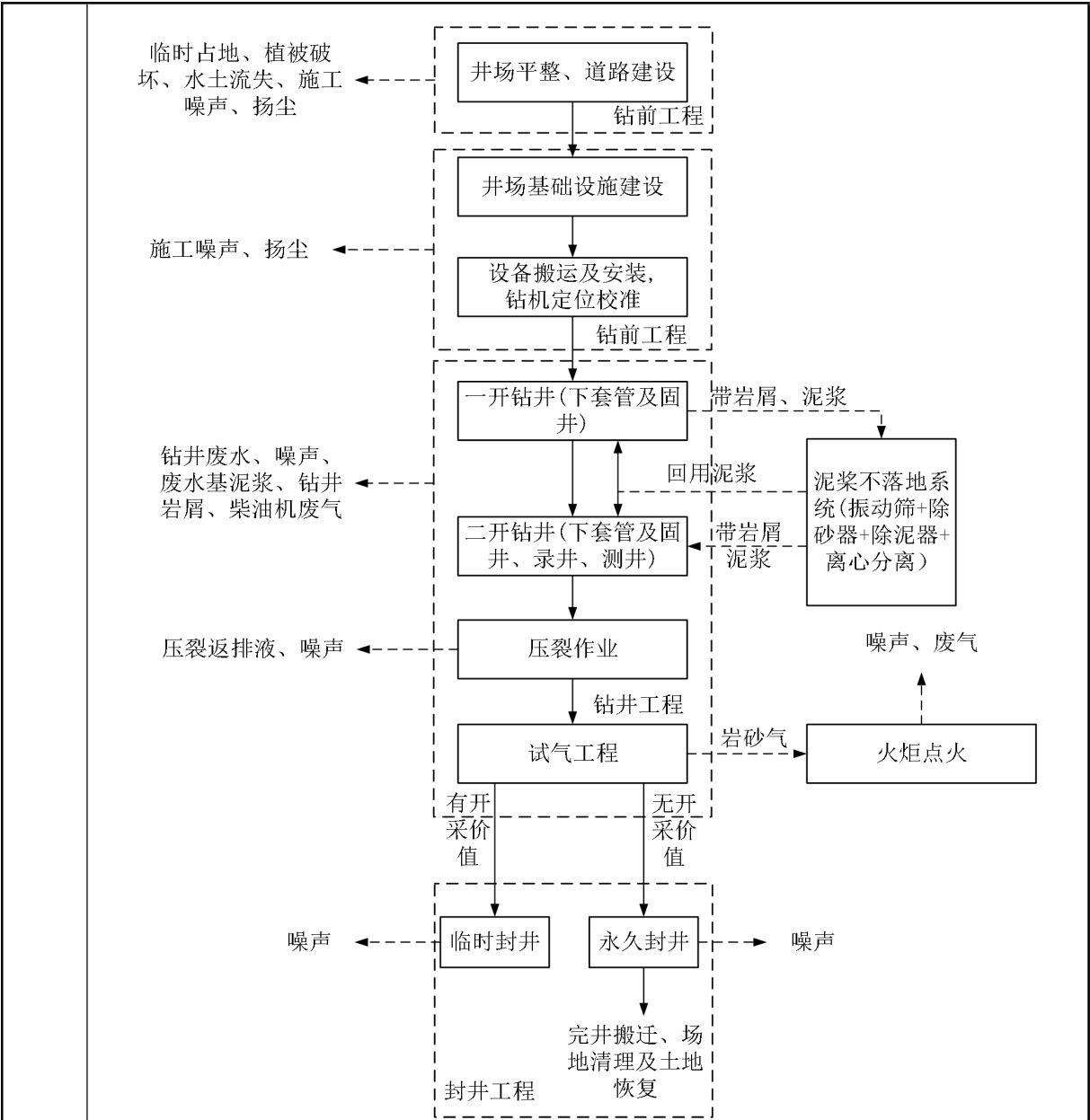
图 2-4 探井工艺流程及产污环节图
