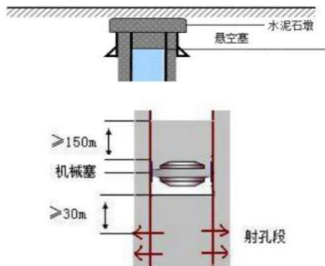
图 2-7 井口及射孔封堵示意图
