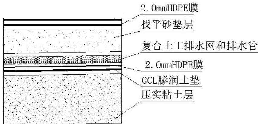
图 5-2 重点防渗区防渗结构示意图
