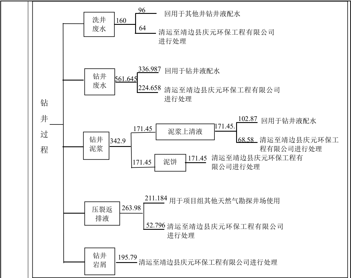
图 2-2 泥饼、岩屑、泥浆、压裂返排液、洗井废水、钻井废水、上清液去向示意图 单位 m³
