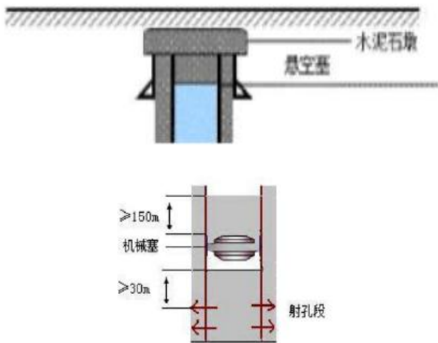
图 2-5 井口及射孔封堵示意图
