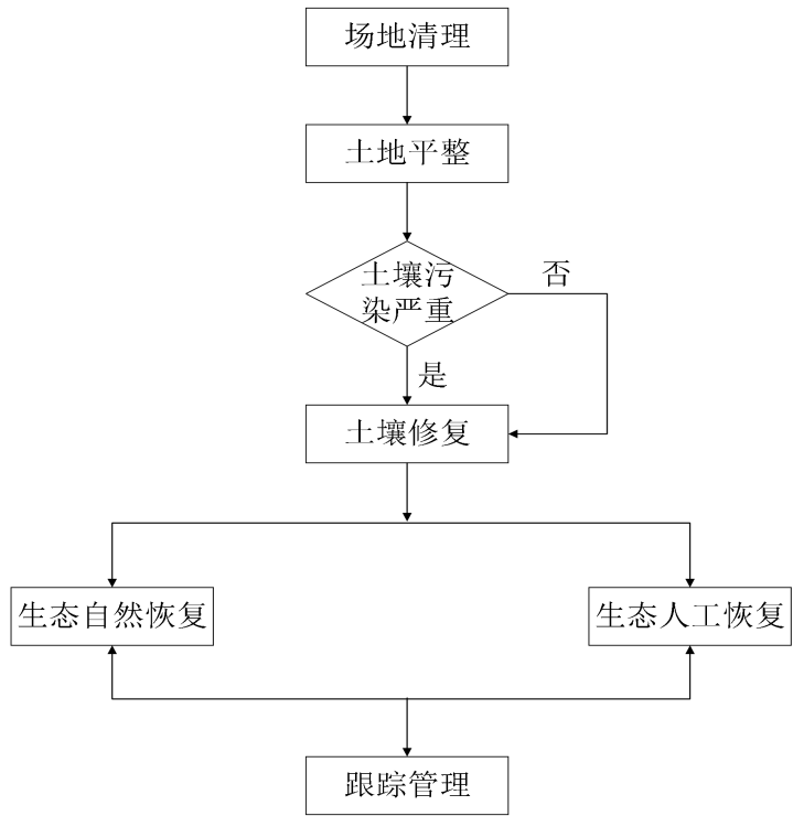
图 5-2 井场生态恢复步骤
