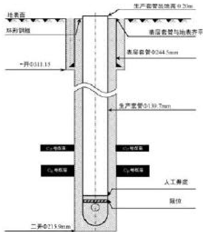
图 2-4 井身结构示意图
