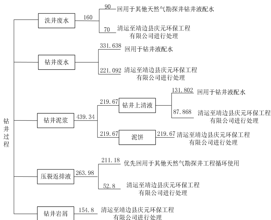
图 2-1 泥饼、岩屑等去向示意图 单位 \text{m}^3
