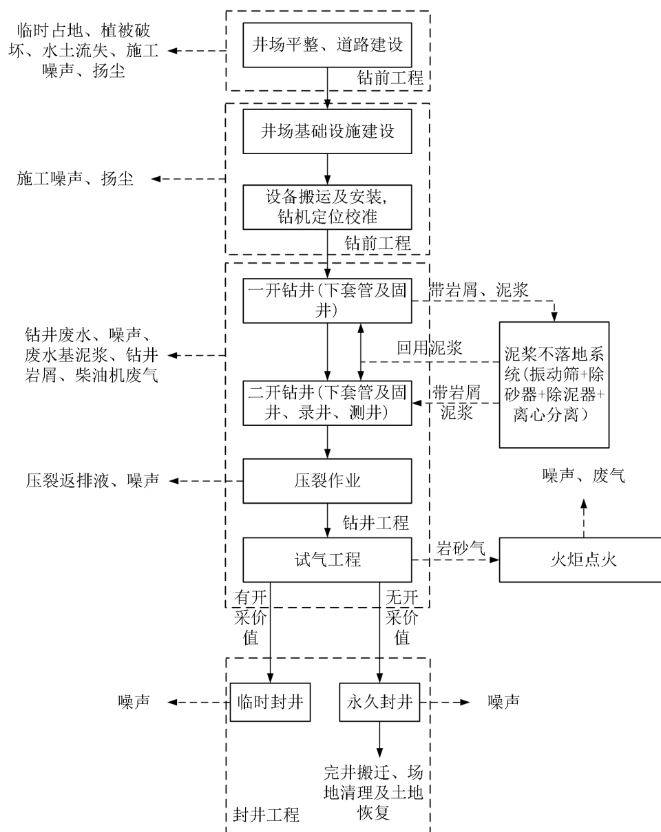
图 2-2 项目主要工艺流程及产污环节图
