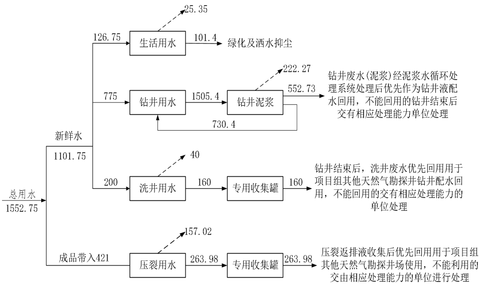
图 2-1 项目水平衡图(单位：m³/65d)
