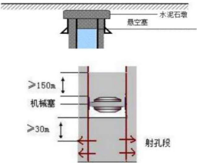
图 2-6 井口及射孔封堵示意图
