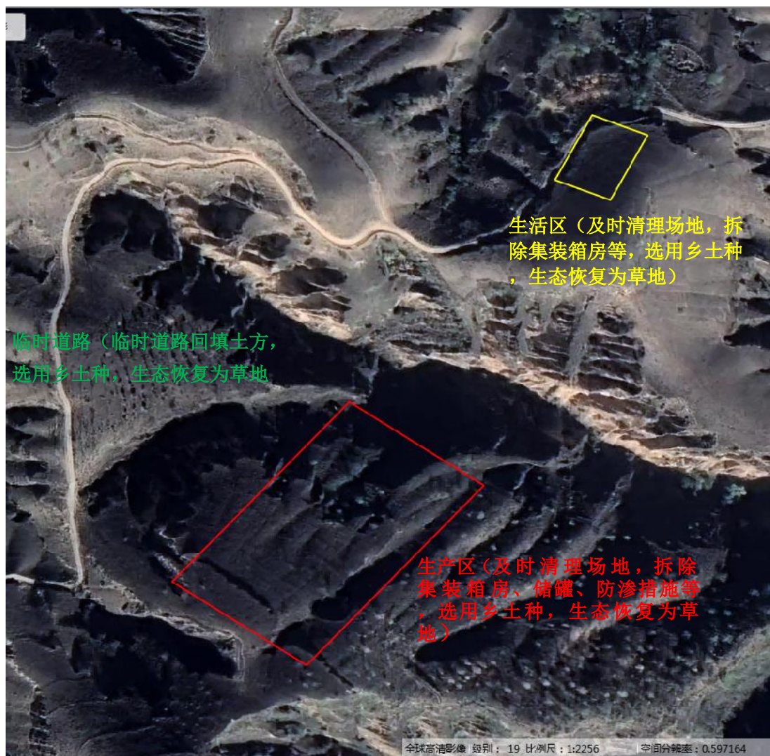
图 5-1 项目生态环境保护措施平面布置示意图
