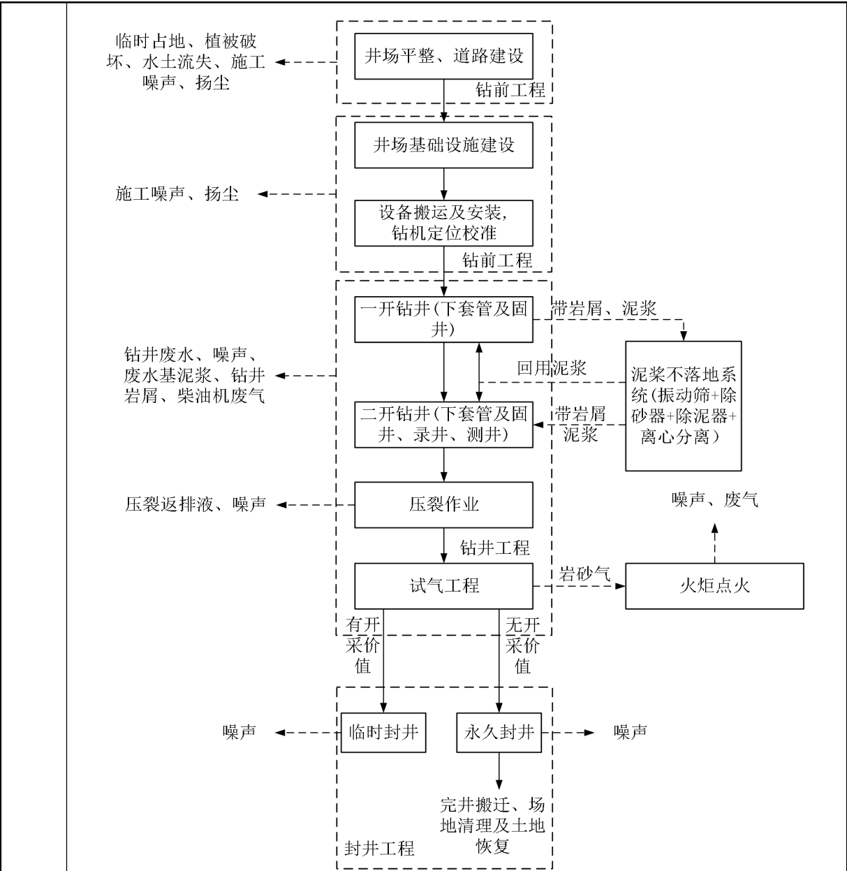
图 2-3 探井工艺流程及产污环节图
