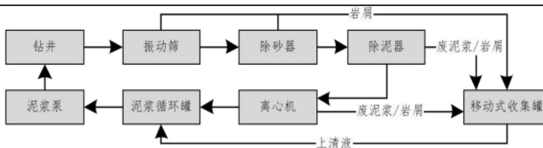
图 2-4 泥浆闭路循环系统示意图
