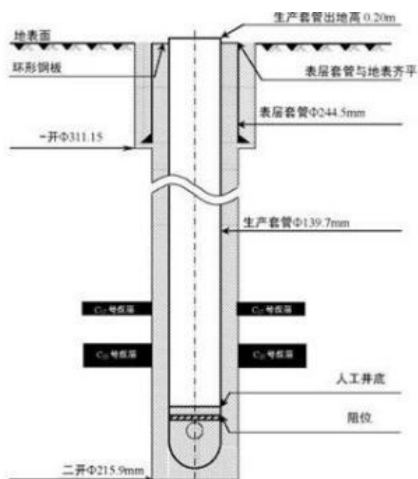
图 2-5 井身结构示意图
